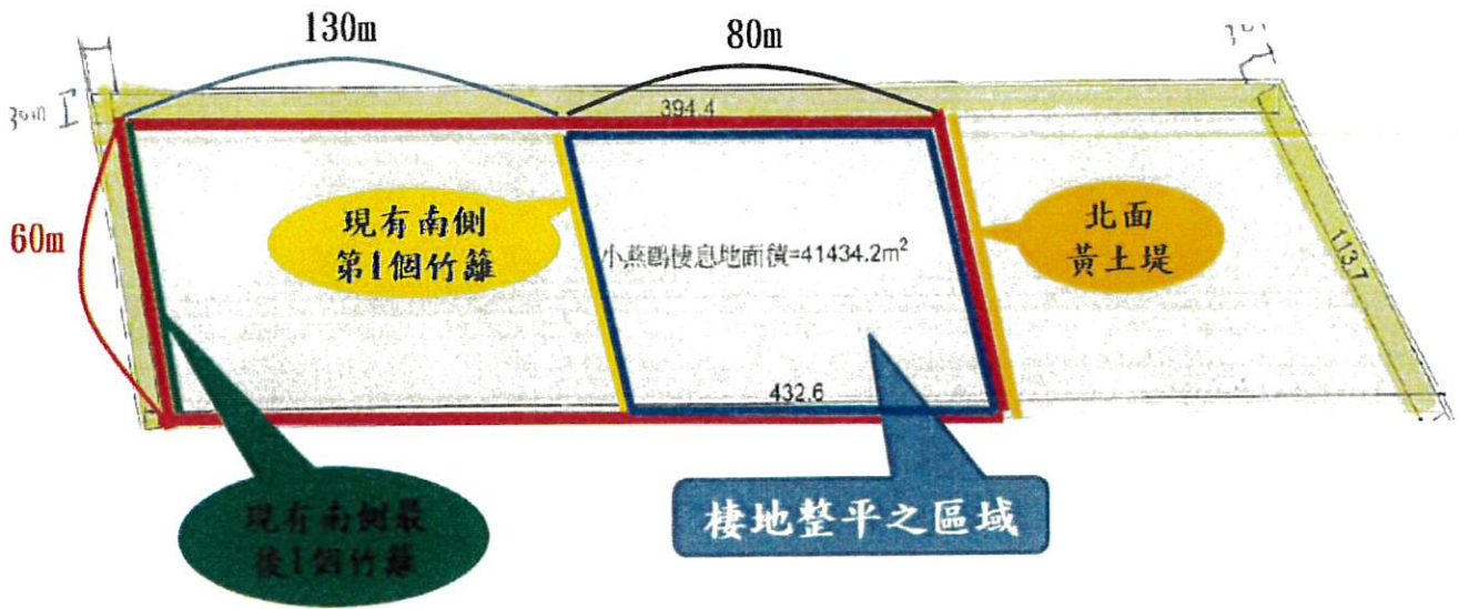
圖(三) 竹圍漁港北岸疏浚用地架設圍籬及棲地整平區域示意圖
